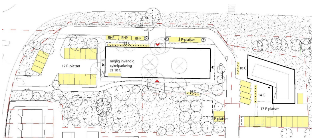
Figuren visar föreslagen parkeringslösning i exploateringsförslaget. (Gaiia arkitektur, Urbio landskapsarkitekter)
