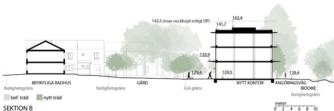
Sektionen genom befintligt radhus, gårdsrummet som bildas och det nya föreslagna kontorshuset. (Gaia arkitektur)
