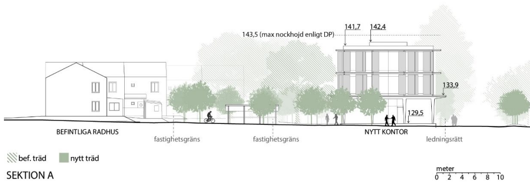
Sektion genom kvarteret, sett från utrymmet mellan det befintliga och nya föreslagna kontorshuset. (Gaia arkitektur)
