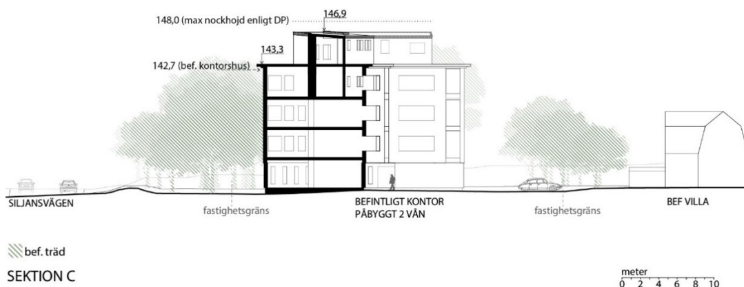
Sektion genom befintligt kontorshus med två möjliga påbyggda våningar i relation till befintligt angränsande bostadshus. Den översta våningen är indragen. (Gaia arkitektur)
