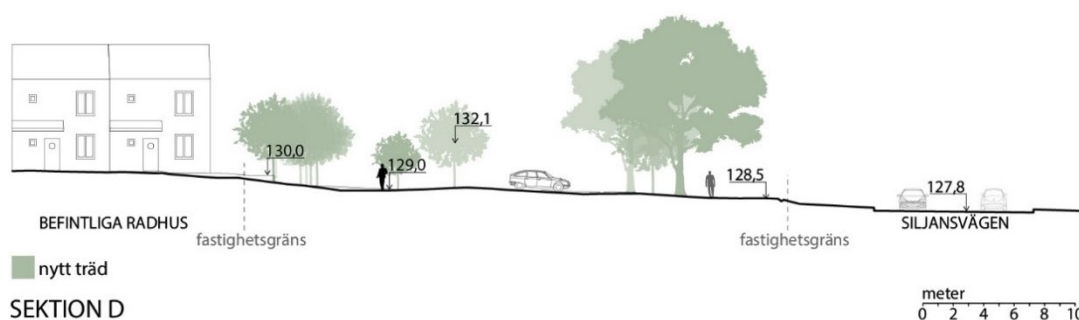
Sektion genom kvarterets norra del, i relation till befintliga radhus. (Gaia arkitektur)
